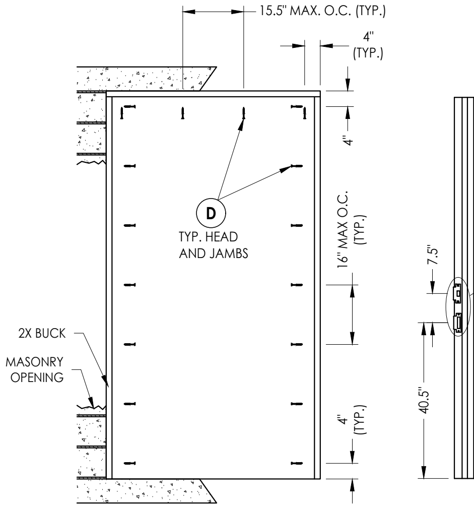
STRIKE JAMB
